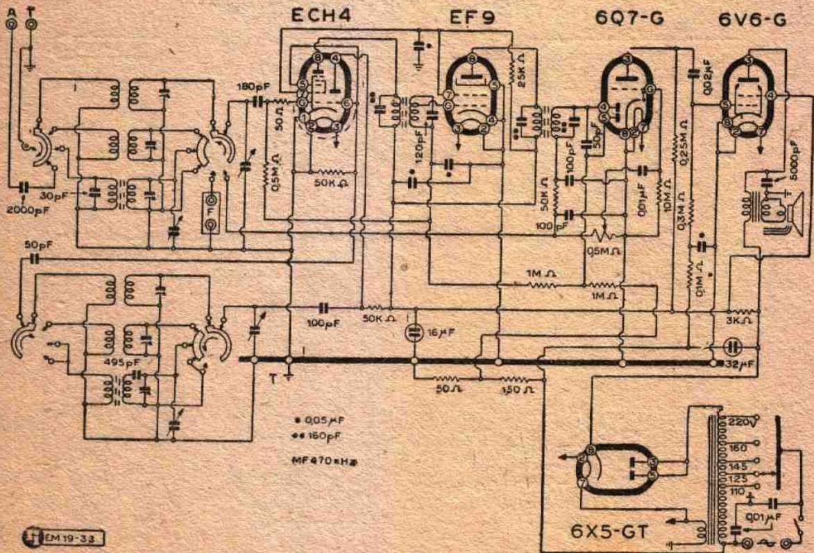
Lo schema elettrico del Minerva mod. "475/5".
