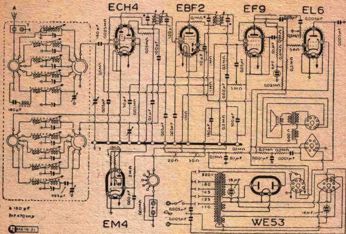
Lo schema elettrico del Minerva mod. "475/1 - Florida".
